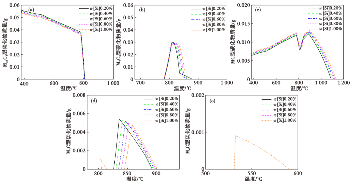
图2 不同Si含量H13钢中碳化物的平衡相图:(a) M 23 C 6 ,(b) M 7 C 3 ,(c) MC,(d) M 2 C,(e) M 6 C
