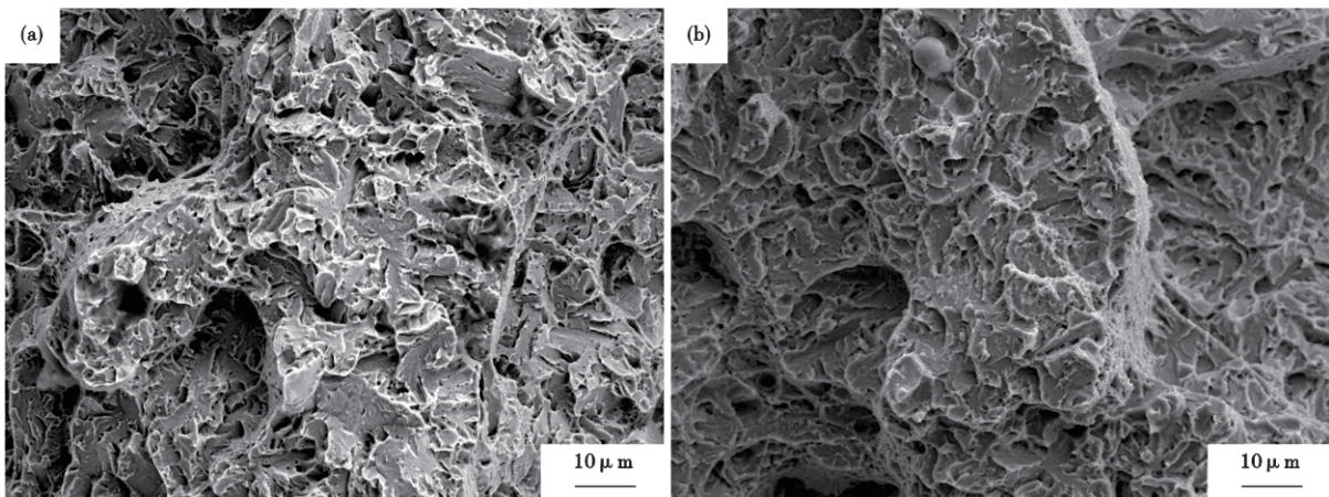
图9 实验钢580 °C回火后的冲击断口形貌:(a) H13钢,(b) DPG20钢
