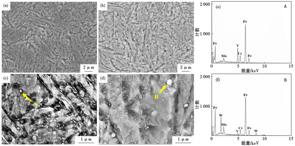
图 10 实验钢的微观组织:(a)(c) H13 钢;(b)(d) DPG20 钢;(e) 碳化物在 A 点的 EDS 能谱图;(f) 碳化物在 B 点的 EDS 能谱图 Fig. 10 Microstructure of experimental steels : (a)(c) H13 steel; (b)(d) DPG20 steel; (e) EDS energy spectrum of carbide at point A; (f) EDS energy spectrum of carbide at point B
